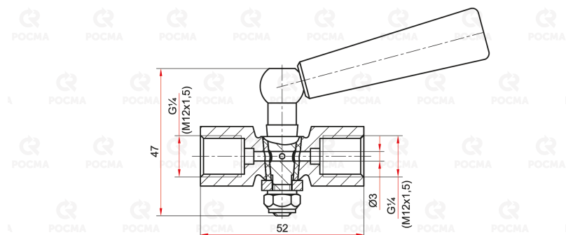
Трехходовой кран с резьбой присоединения G\frac{1}{4} или M12x1.5
