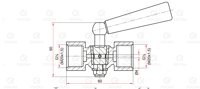
Трехходовой кран с резьбой присоединения G\frac{1}{2} или M20x1,5
